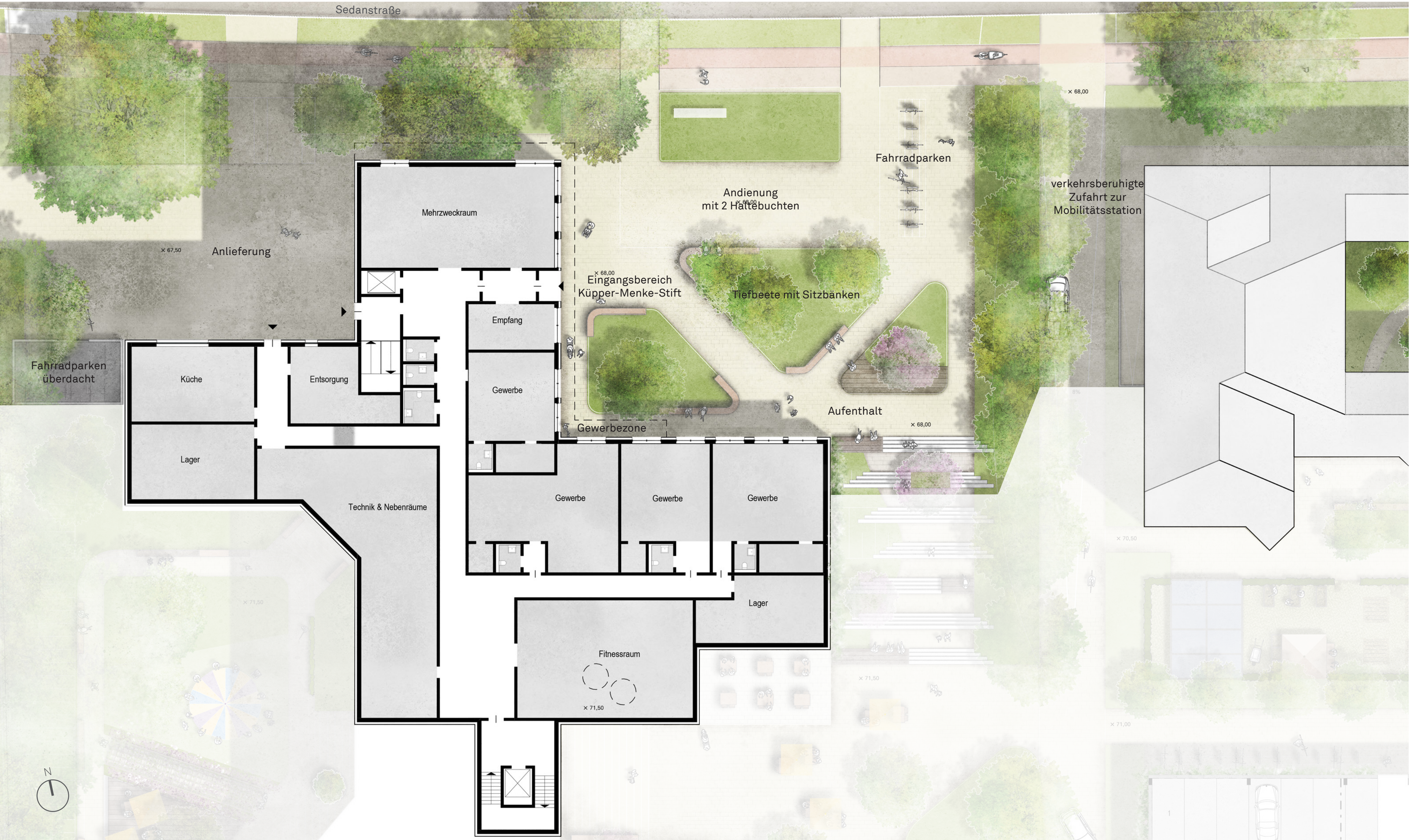
Lageplan M 1:200 | Ebene Entrée und Anlieferung
